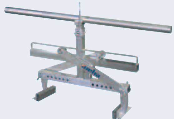
Treppenstufenzange Stair Tread Tong Art.-# VD080507
